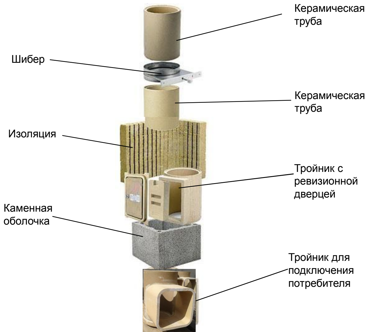
Дымоходная система UNI для печей Скандинавского типа.
