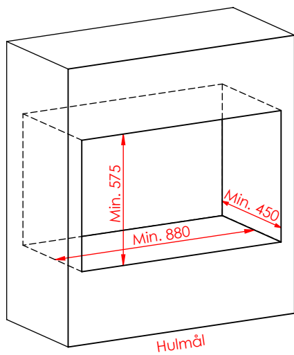
JUPITER 550 - 850, FRISKLIFT BAG.
