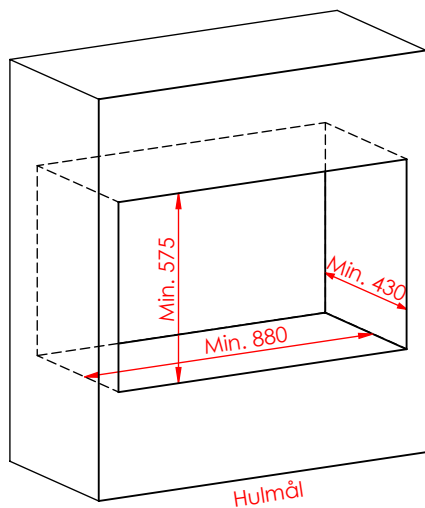
JUPITER 550 - 850, FRISKLIFT TOP.
