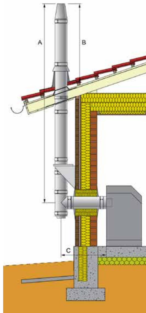
ICS25 modulūdūmvada savienošana ar apkures iekārtu. Zīmējums ir ilustratīvs.
