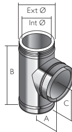
93° Tee
