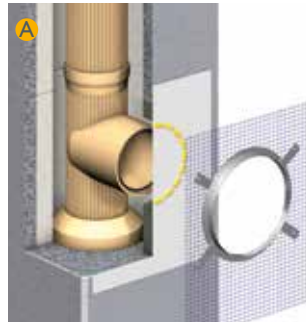
Blower-Door-dichter Rauchrohr-Anschluss
