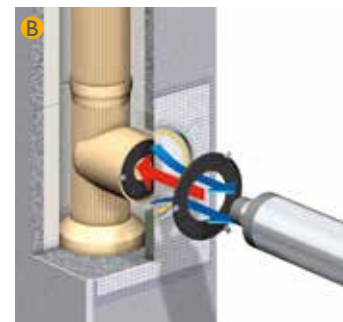
Steck-Adapter innen und außen Ringspalt nur bei li. \varnothing 12+14 \text{ cm}
