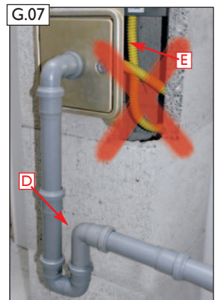
Ableitung mit HT-Rohren DN40 mit Aufweitungen zum Bodenablauf vor dem Schornstein.
