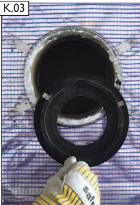
Steckadapter laut beiliegender Anleitung einsetzen. (Sonderzubehör; bitte extra bestellen!) Verbindungsleitung in Steckadapter einbringen.
