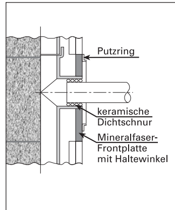
Standardanschluß für Öl- und Festbrennstoffkessel Ringspalt zwischen Schamottestutzen und Rauchrohr mit keramischer Schnur abdichten. Auf freie Beweglichkeit des Feuerstättenanschlusses achten!
