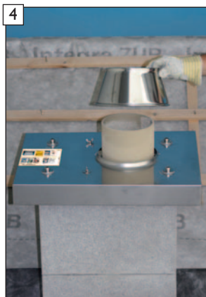
Konus aufstecken. WICHTIG! Oberkante Konus muss auf dem Keramikrohr aufliegen!
