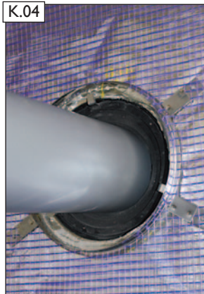
Steckadapter laut beiliegender Anleitung einsetzen. (Sonderzubehör; bitte extra bestellen!) Verbindungsleitung in Steckadapter einbringen.
