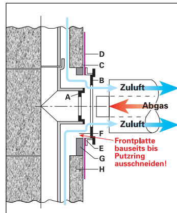
Standardanschluß für Gas/Brennwertkessel (max. Anwendungstemperatur 200^{\circ}\text{C} ) Steckadapter nach Einbauhinweis einsetzen.
