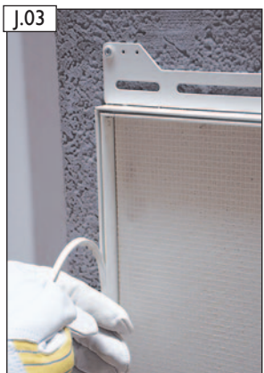
J.03 Schutzdichtung in den Türspalt der BlowerDoor Design-Putztür einbringen und an der Ecke abschneiden.
