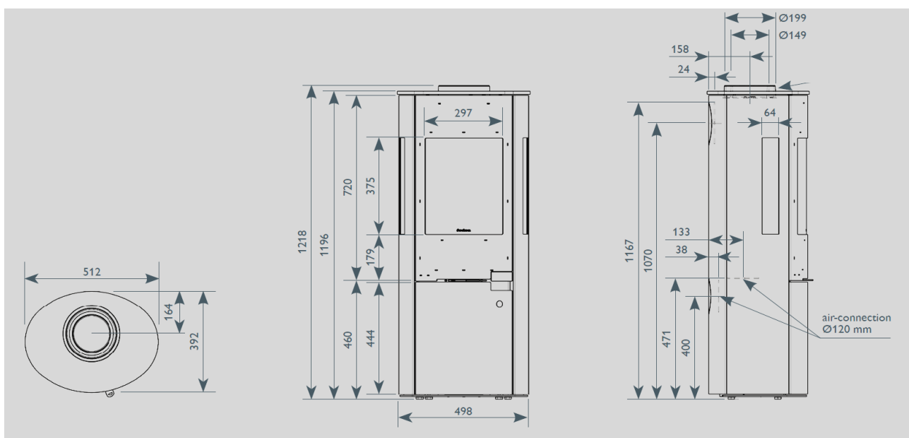
ANSICHT VON OBEN
